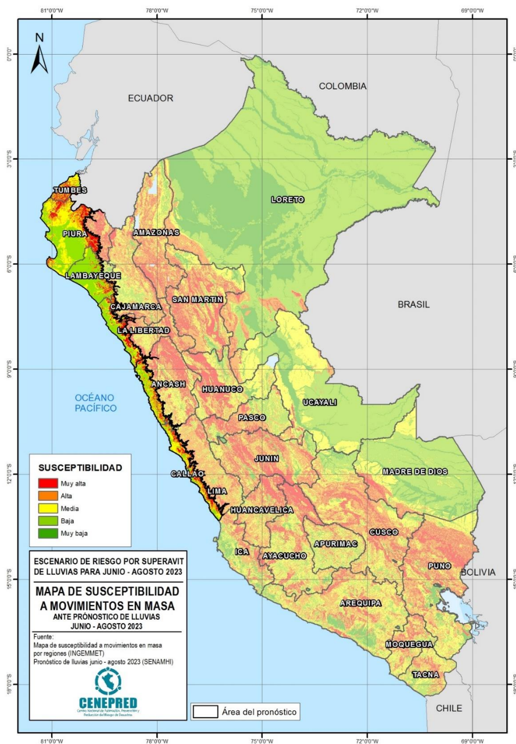
Figura 7. Mapa de susceptibilidad por movimientos en masa ante el pronóstico de lluvias para junio – agosto 2023
