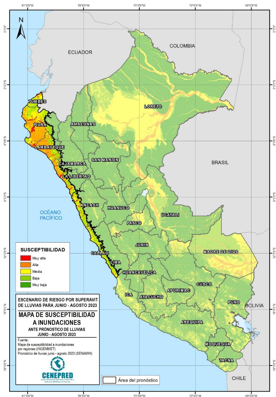
Figura 9. Mapa de susceptibilidad a inundaciones ante el pronóstico de lluvias para junio - agosto 2023
